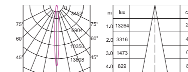
TL-MS76 15W 4000K CRI>90 15°
