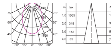
TL-MGL640 20W 4000K CRI>90 110°
