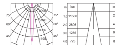
TL-MS76 15W 3000K CRI>90 15°
