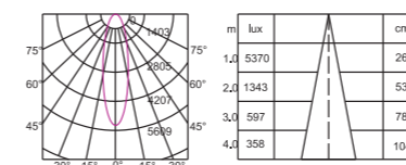
TL-MLS10 10W 3000K CRI>90 30°
